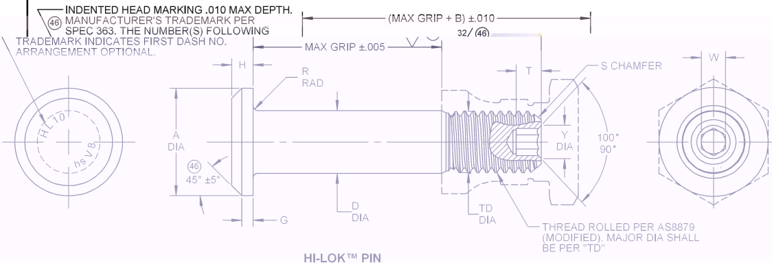
HI-LOK™ PIN
