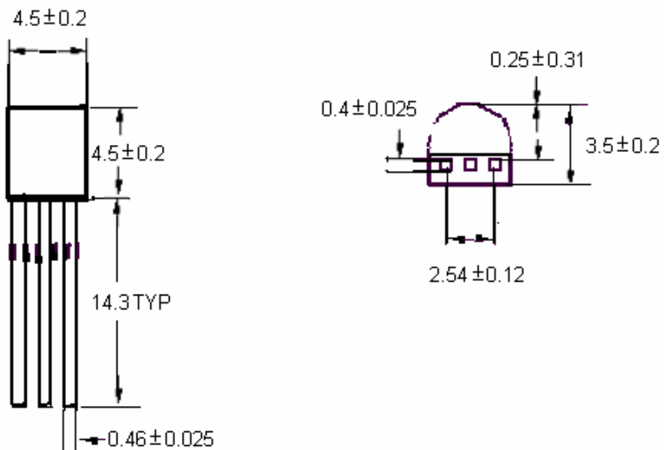
TO-92 Unit:mm
