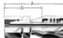
Metric universal female swivel 60° DIN 7631/7647 07.002-/07.036-
