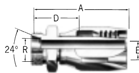
Metric male 24° DIN 3901/3902 I.Rh. 07.003-
